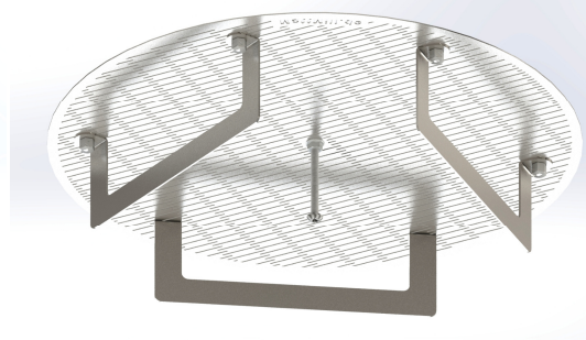
Fertig montiert Ansicht Unterseite
